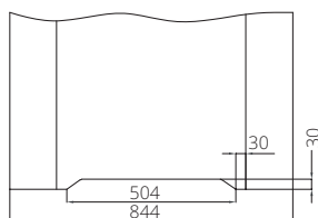
křídlo „80“ s ventilačním seříznutím
