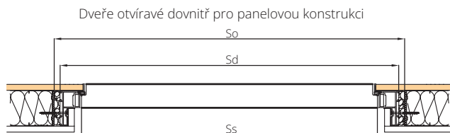
DRZWI OTWIERANE DO WEWNĄTRZ ODW
