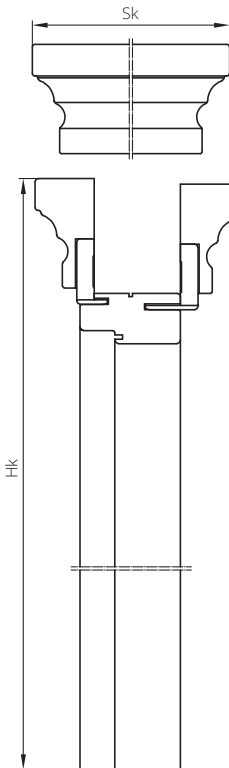
Sk – šířka na vnější straně korunky Hk – výška na vnější straně korunky
