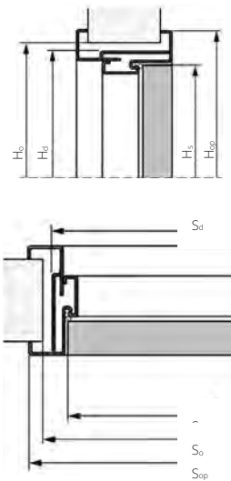
EI30 PLUS, EI60 PLUS ZÁRUBEŇ KOVOVÁ NASTAVITELNÁ
