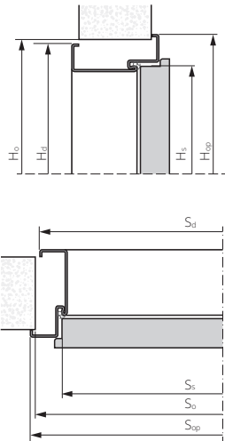
EI30 PLUS, EI60 PLUS, RC3, GAMMA, DECO INVEST, CERBER PLUS ZÁRUBEŇ KOVOVÁ PEVNÁ
