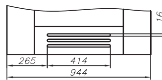
křídlo „90“ s ventilační štěrbinou
