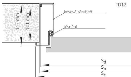
PEVNÁ KOVOVÁ SYSTÉM POL-SKONE FD12:
