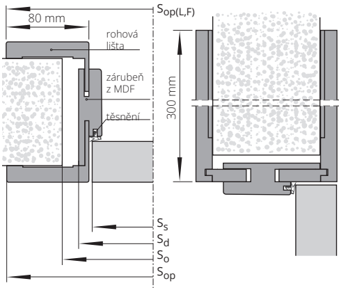
NASTAVITELNÁ BEZFALCOVÁ SYSTÉM VERTIGO:
