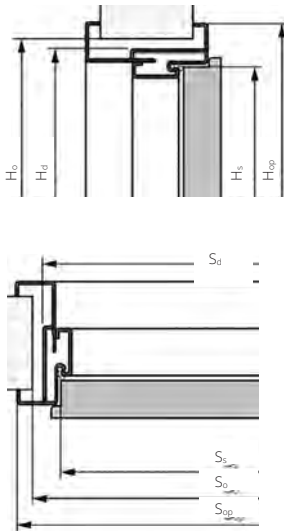
DVEŘE KYVNÉ ZÁRUBEŇ DŘEVĚNÁ PEVNÁ
