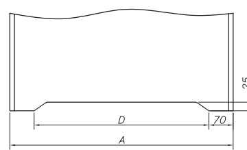
ventilační seříznutí ve falcových křídlech - příplatek dýhované povrchy •/• - příplatek syntetické/stříkané povrchy •/•
