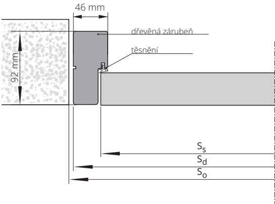
PEVNÁ BEZFALCOVÁ DUO:
