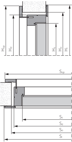
EI30 PLUS, EI60 PLUS ZÁRUBEŇ KOVOVÁ NASTAVITELNÁ
