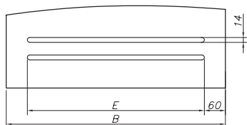
ventilační štěrbinu v bezfalcových křídlech
