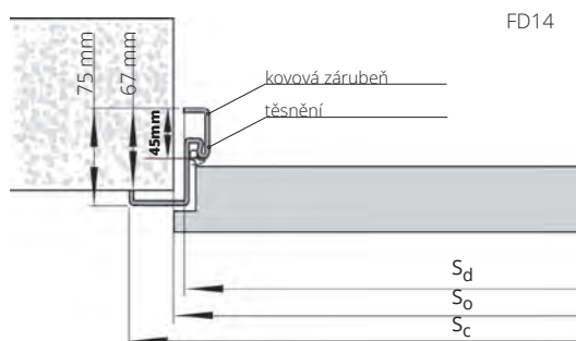
PEVNÁ KOVOVÁ SYSTÉM POL-SKONE FD14:
