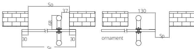
Dveře levé s podélným madlem
