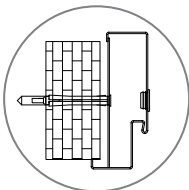
montážní otvor na kotvu ve středu profilu na čele zárubně
