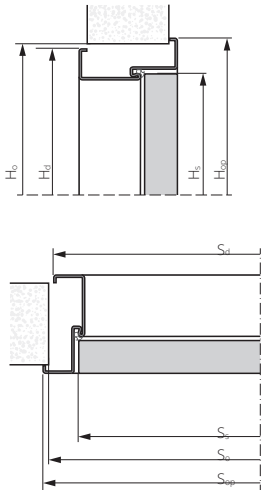
EI30 PLUS, EI60 PLUS, HIGRO ZÁRUBEŇ KOVOVÁ PEVNÁ
