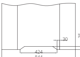
křídlo „80“ s ventilačním seříznutím
