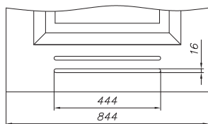
křídlo „80“ s ventilační štěrbinou
