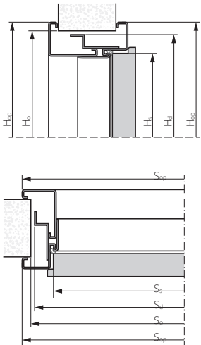
ZVUKOTĚSNÉ TYP A, B, DECO INVEST, GAMMA ZÁRUBEŇ KOVOVÁ NASTAVITELNÁ
