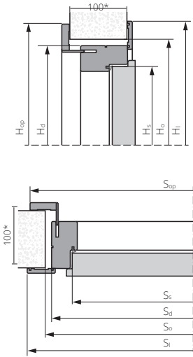
FR EI30, EI 30 PLUS, EI 60 PLUS, B-30, C-30, RC3, SR 37 dB, SR 42 dB, CERBER PLUS, GAMMA ZÁRUBEŇ DŘEVĚNÁ
