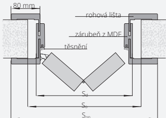
nastavitelná DIN DUO
