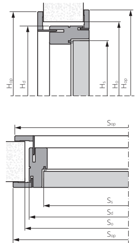
ZVUKOTĚSNÉ TYP A, B ZÁRUBEŇ DŘEVĚNÁ BEZFALCOVÁ
