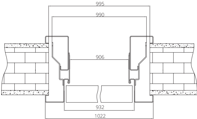
Nastavitelná kovová zárubeň šíř. „90“
