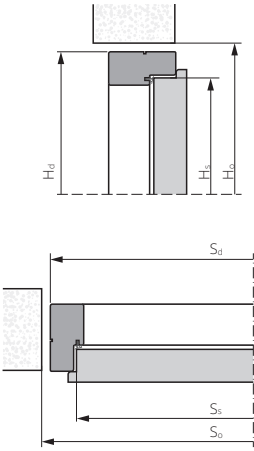
ZVUKOTĚSNÉ TYP A, B ZÁRUBEŇ DŘEVĚNÁ PEVNÁ
