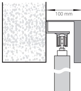
nástěnný posuvný systém s tunelovou zárubní ZN (neplatí pro systém PREMIUM)
