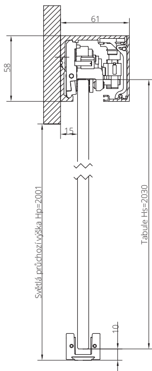
Dveře levé s podélným madlem
