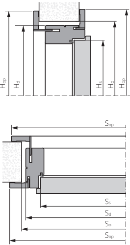
ZVUKOTĚSNÉ TYP A, B ZÁRUBEŇ DIN ZP NASTAVITELNÁ
