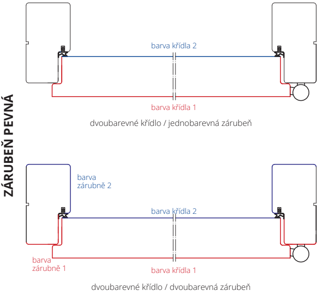
dvoubarevné křídlo, jednobarevná zárubeň
