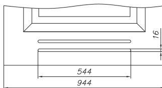
křídlo „90“ s ventilační štěrbinou
