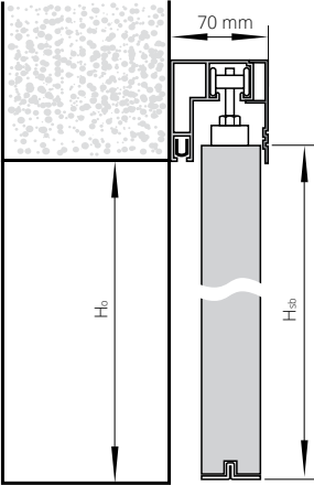
DÉLKY KRYCÍCH LIŠŤ PRO SYSTÉM NÁSTĚNNÝ PREMIUM
