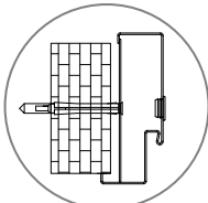
montážní otvor pro kotvu ve středu profilu na čele zárubně
