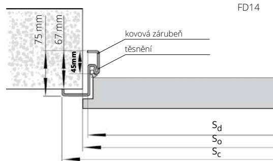
PEVNÁ KOVOVÁ SYSTÉM POL-SKONE FD14:
