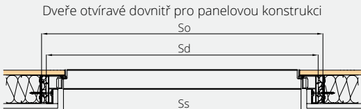
Dveře otvíravé dovnitř pro panelovou konstrukci
