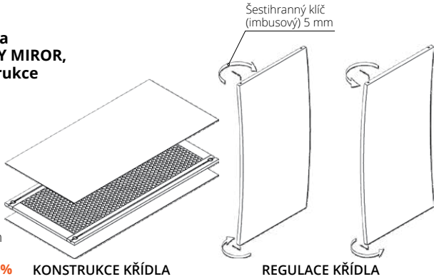
KONSTRUKCE KŘÍDLA
