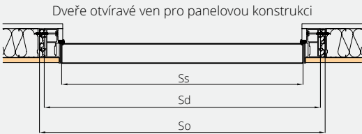
Dveře otvíravé ven pro panelovou konstrukci
