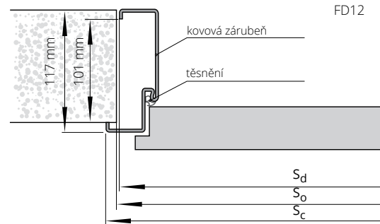
PEVNÁ KOVOVÁ SYSTÉM POL-SKONE FD12:
