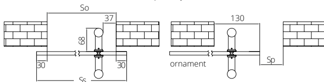
Levé dveře s podélným madlem
