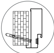
montážní otvor pro kotvu ve falcí zárubně
