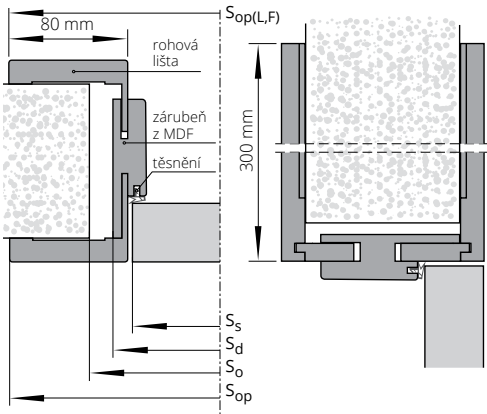
NASTAVITELNÁ BEZFALCOVÁ SYSTEM VERTIGO:
