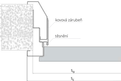
NASTAVITELNÁ KOVOVÁ DIAGONAL SYSTÉM POL-SKONE:
