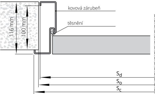
PEVNÁ KOVOVÁ DUO SYSTÉM POL-SKONE:
