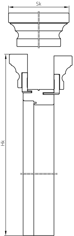
Sk – šířka po vnější straně korunky Hk – výška po vnější straně korunky
