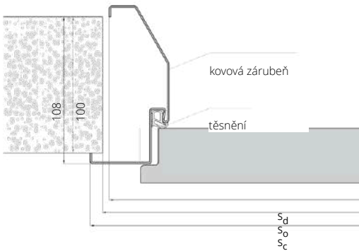
PEVNÁ KOVOVÁ DIAGONAL SYSTÉM POL-SKONE:
