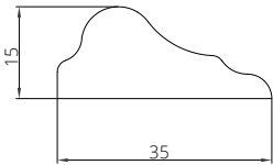
Průřez profilu dekorativní lišty
