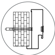
montážní otvor kotvy ve středu profilu na čele zárubně
