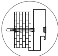
montážní otvor na kotvu ve středu profilu na na čele zárubně
