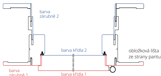
dvoubarevné křídlo / dvoubarevná zárubeň
