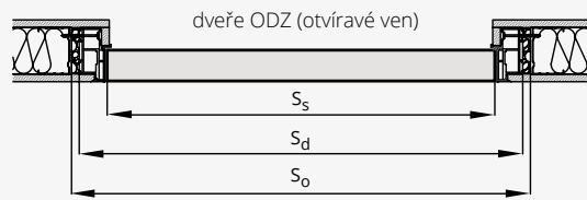
DVEŘE OTVÍRÁVÉ VEN ODZ
