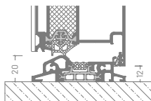
Bezbariérový práh s přerušeným tepelným mostem do výšky 20 mm
